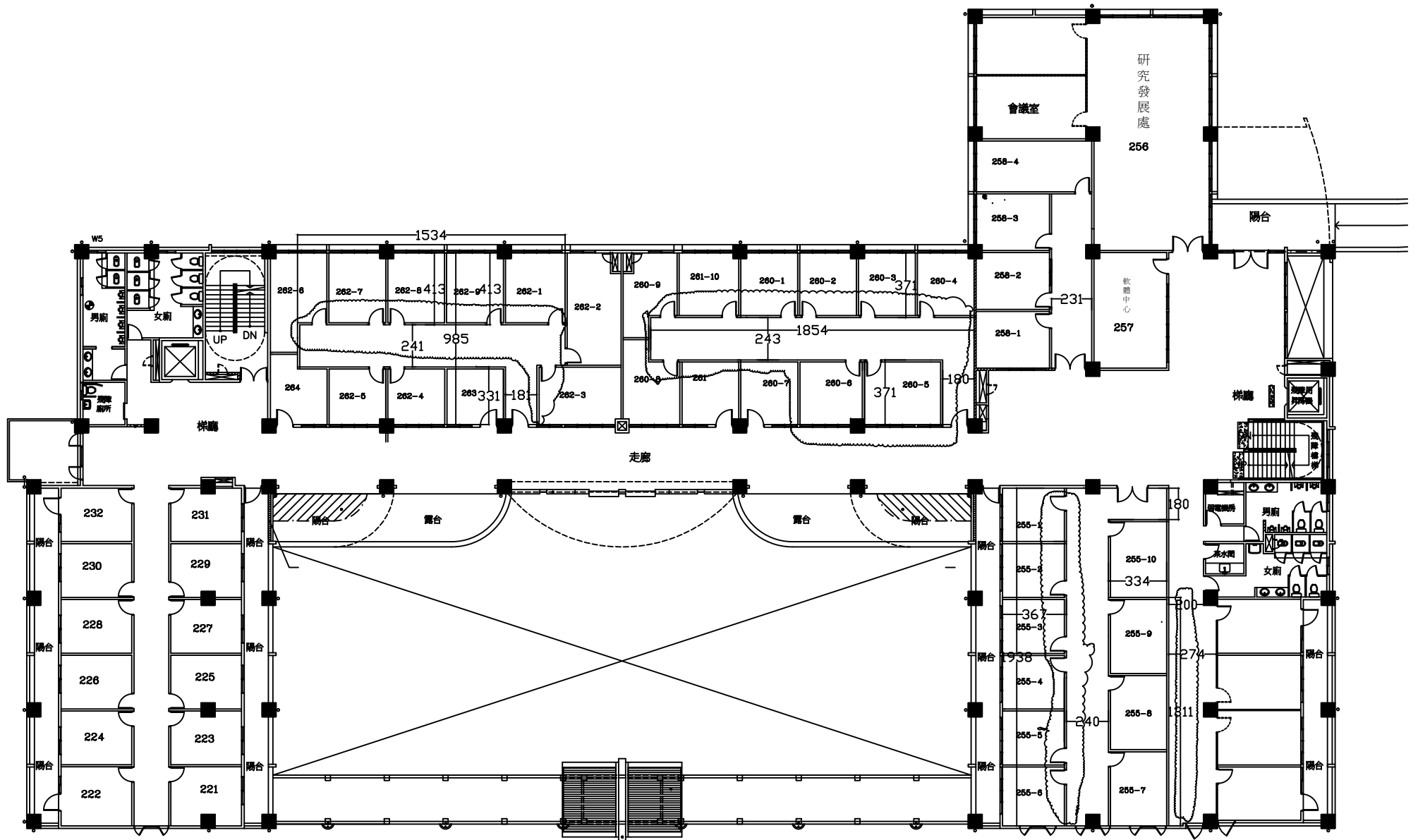
智耕樓二樓平面圖
